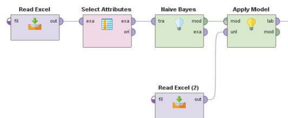
Gambar.4.3.1. Proses Pengujian Rapid Miner
