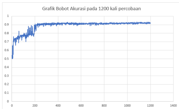
Gambar 20. Bobot Akurasi
