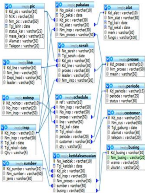
Gambar 7.. Relasi Antar Tabel
